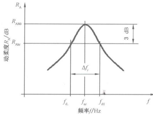
图4 动柔度曲线中第 i 阶共振峰的半功率带宽
